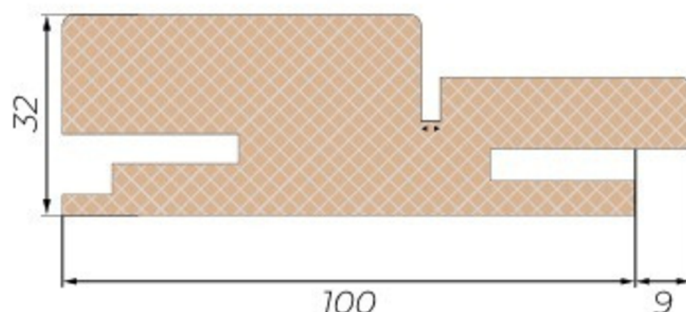
DETALIU TOC REGLABIL MDF 10X32X2050
