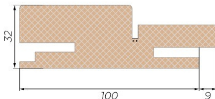
DETALIU TOC REGLABIL MDF 10X32X2050
